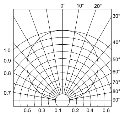
Radiation Diagram 辐射特性曲线
