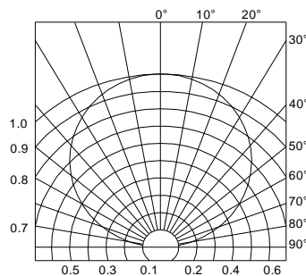
Radiation Diagram 辐射特性曲线
