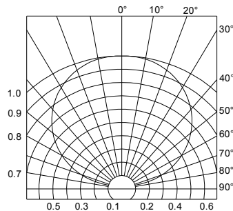
Radiation Diagram 辐射特性曲线
