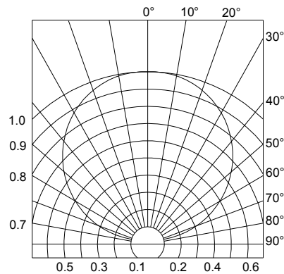
Radiation Diagram 辐射特性曲线
