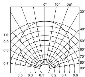
Radiation Diagram 辐射特性曲线
