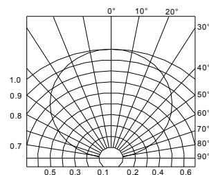
Radiation Diagram 辐射特性曲线
