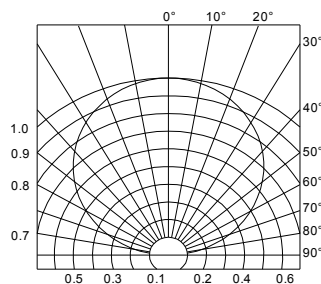
Radiation Diagram 辐射特性曲线
